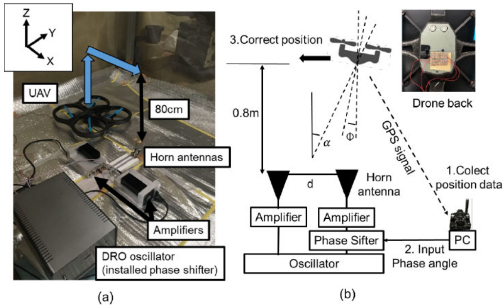
図 電波シールドルーム内でのマイクロ波ワイヤレス給電実験
