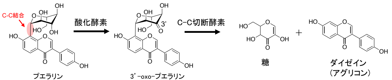
図2 プエラリンの C-C 結合切断反応
