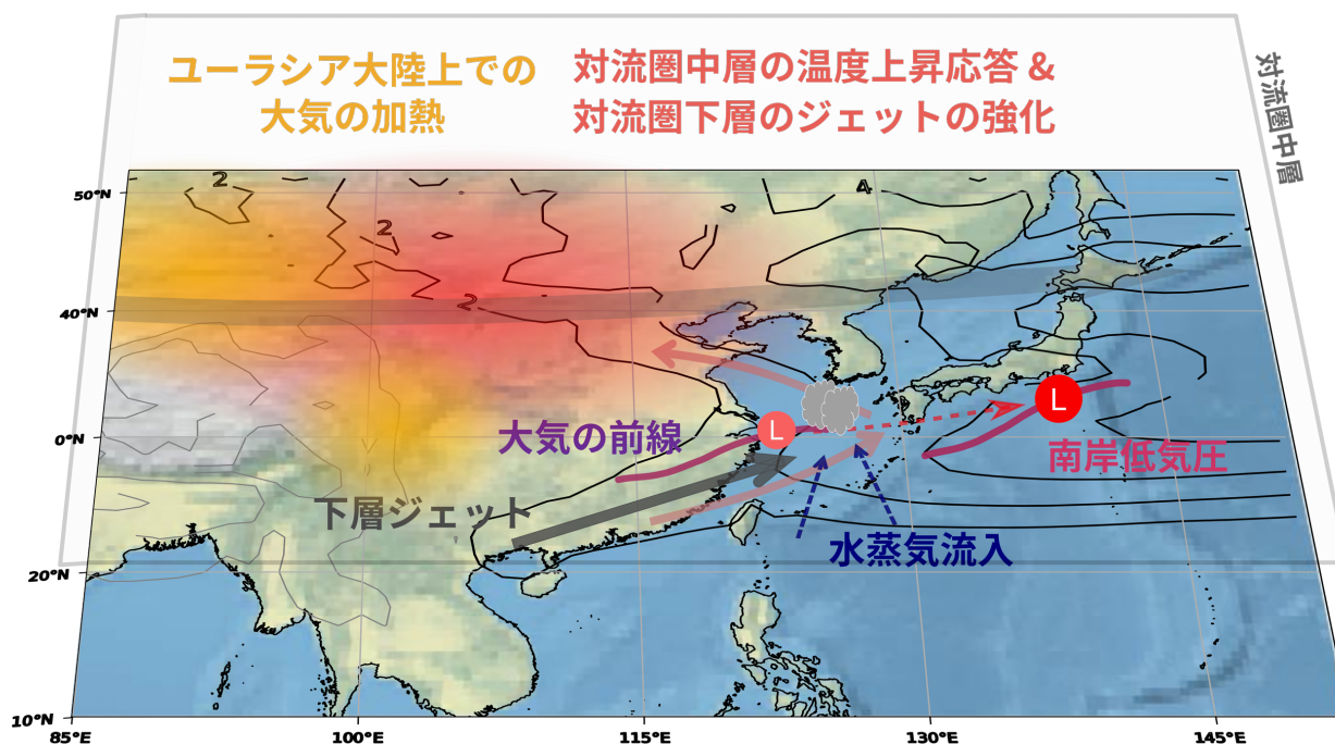
図 本研究で明らかになった南岸低気圧活動の春のピークのメカニズム
