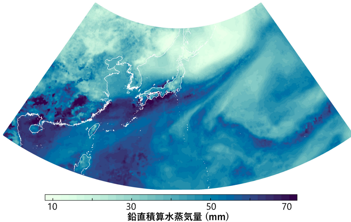
図1 大気の水蒸気が日本列島周辺を通過する様子 令和2年7月豪雨発生時の大気中の水蒸気量の分布。水蒸気が大量に流れる「大気の水蒸気」が東西に長く伸び、中国長江流域や西日本、東日本上空を流れている。
