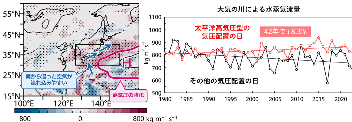
図2 日本列島周辺を流れる大気の水蒸気による水蒸気流量の変化傾向 「太平洋高気圧型」の日を対象に、大気の水蒸気による水蒸気流量を分析して得られた変化傾向。地球温暖化による全体的な水蒸気量の増加傾向に加え、太平洋高気圧が強まることで（左図）、その西縁を北上する水蒸気の流れが強まっている（右図）。
